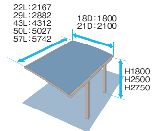
Mini
